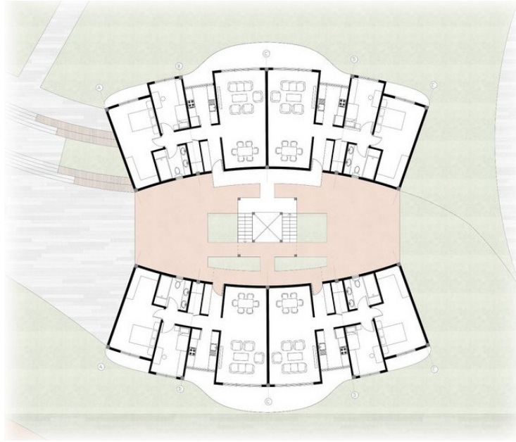
Tip kat planı
