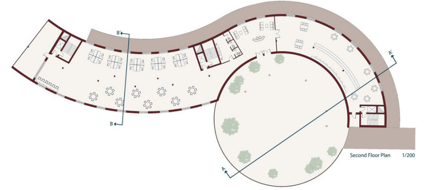
02 / İkinci kat planı
