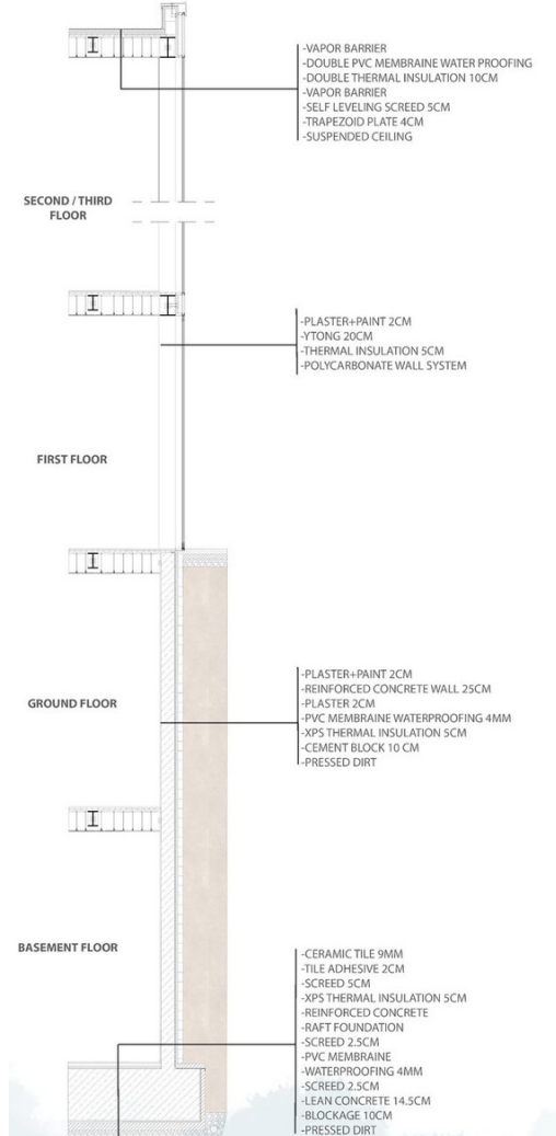
01 / Yapı kesiti
