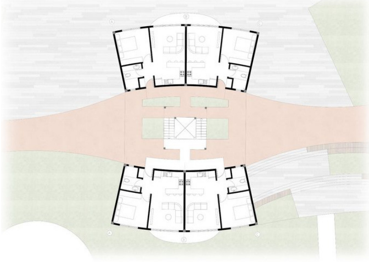
Tip kat planı
