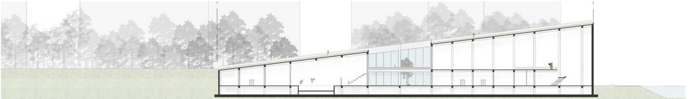
03 / Section A-A
